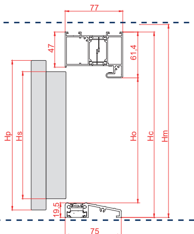
DUOTHERM 75
