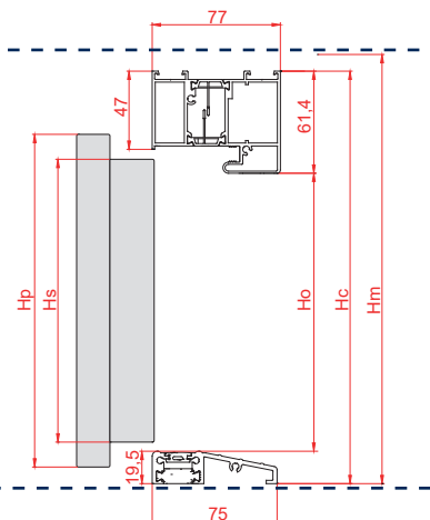
DUOTHERM 60
