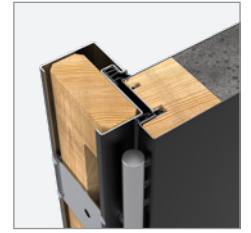
Ościeżnica DUOTHERM 60
